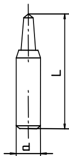
WD3 mit Körner-Spitze 70°
