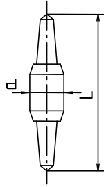
WD3 mit Körner-Spitze 70°
