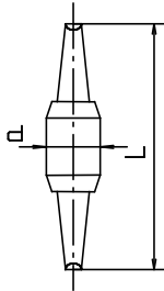
WD4 mit eingekerbter Spitze
